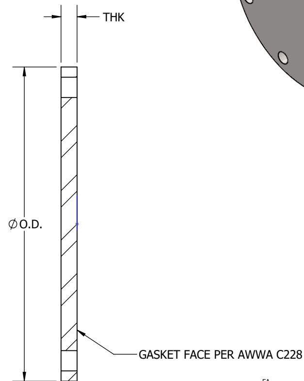
SECTION A-A
